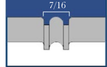
Mini V-Groove
