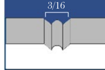
V-Groove
